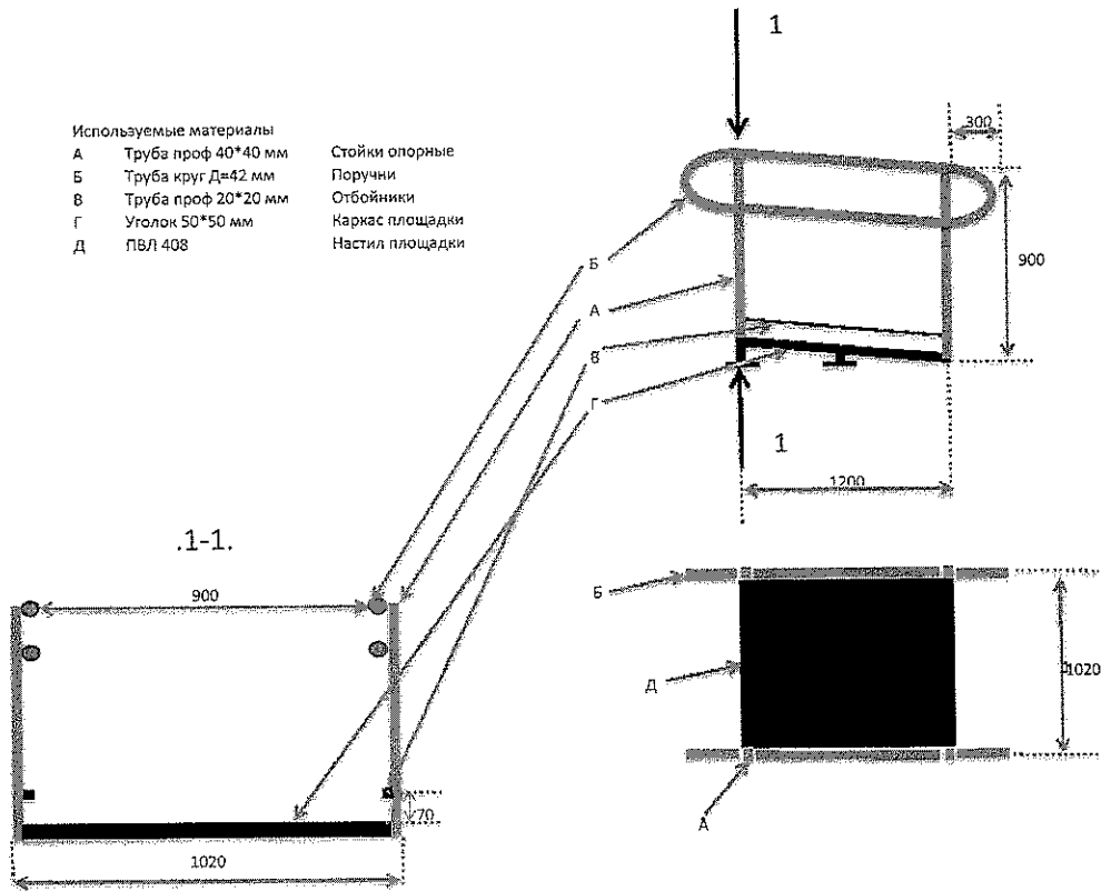
Эскизный чертеж Пандуса
